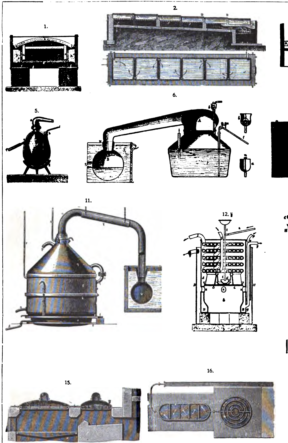
1. Стушение до 60° Б. съ нагрѣвомъ сверху (поперечный разрѣзь) 2. Тоже съ нагрѣвомъ снизу (продольный разрѣзь). 3. Стушение до 60° Б. въ стеклянныхъ ретортахъ. 4. Часть ретортнаго отдѣленія въ планѣ. 5. Сифона Бреанта съ холодильникомъ Либиха (разрѣзь). 6. Плоскій платиновый кубъ Desmoutis Lemaire (Форы и Кесслера въ разрѣзь. 13 и 14. Двойной платиновый аппаратъ системы Дельпласа для стушения. 17. Продолговатый кубъ съ концентрическими перегородками (планъ). 18 и 19. Стушение по способу Л. отъ мышьяка стринстымъ
